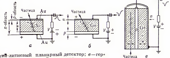
маний-литиевый коаксиальный детектор.
